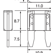
ミニ平型ヒューズ (BFMN)
