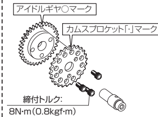
図1：各ギヤの「○」と「・」マークを一致させて取り付けて下さい
