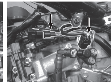
③インジェクター (2P カブラ)
